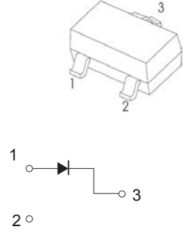
SOT-23
